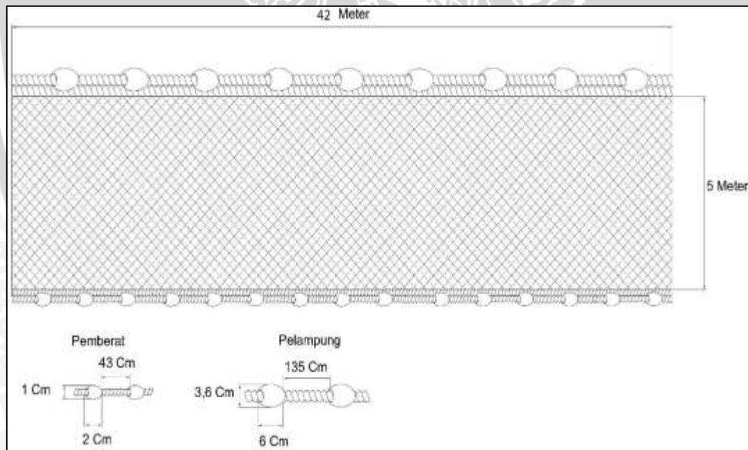
Alat Tangkap Jaring Insang Dasar
