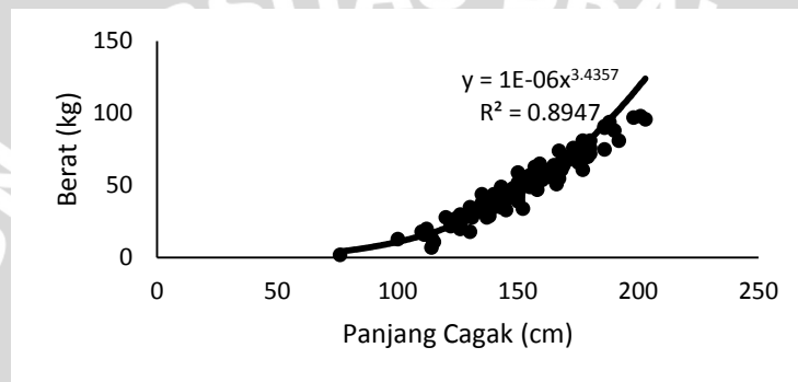
Gambar 26. Hubungan Panjang dan Berat Ikan Hiu Paitan ( Alopias superciliosus )
