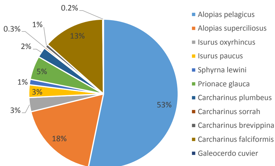
Gambar 23. Komposisi Spesies Hiu Hasil Tangkapan Pancing Rawai
