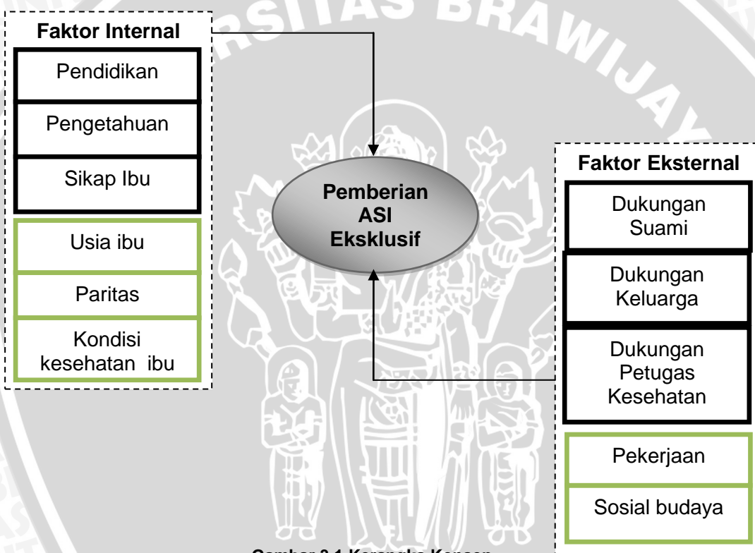
Gambar 3.1 Kerangka Konsep
