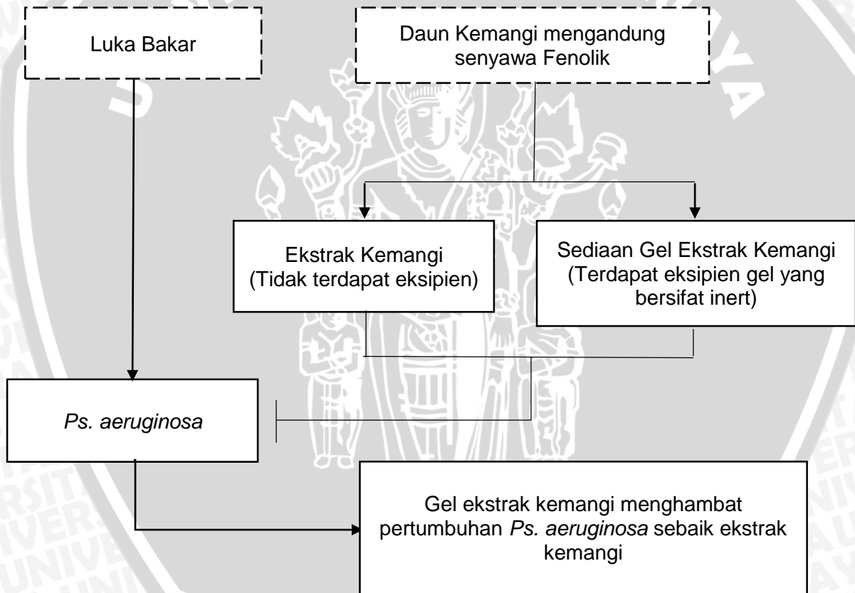
Gambar 3.1 Kerangka Konseptual
