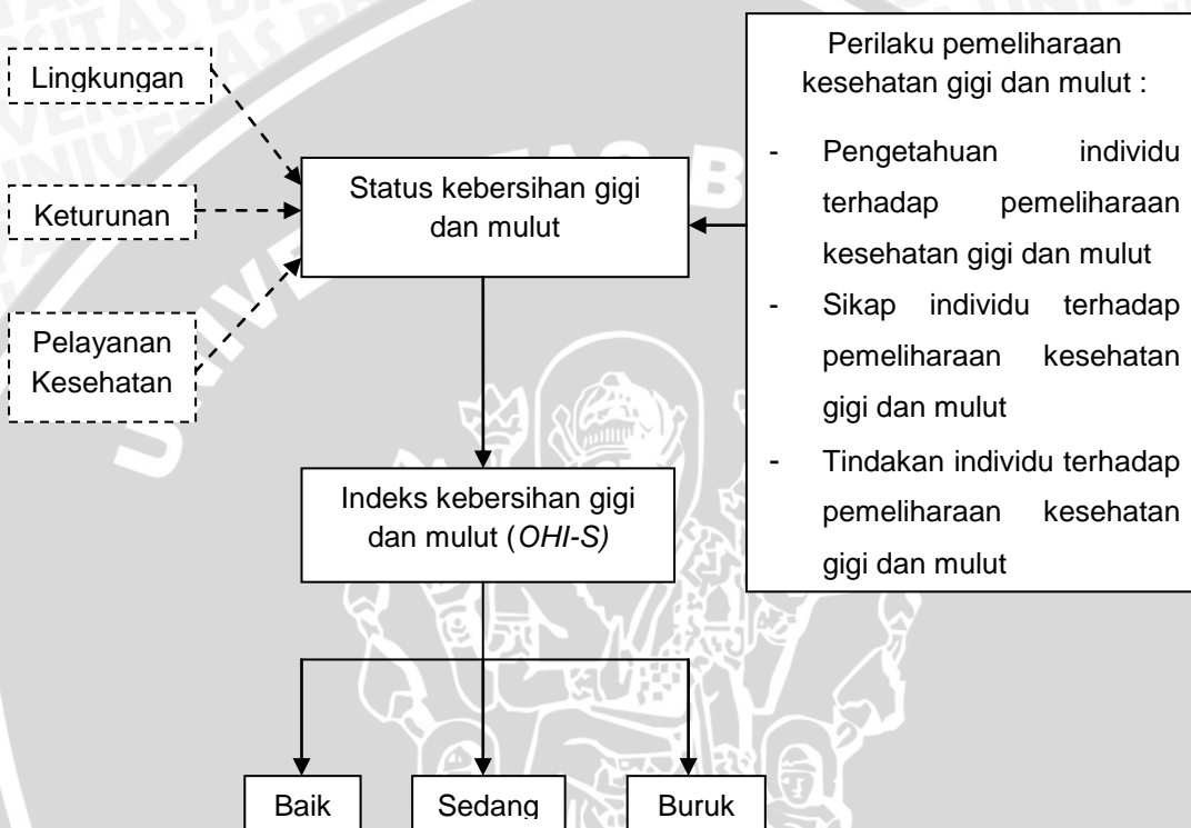
Gambar 3.1 Kerangka Konsep
