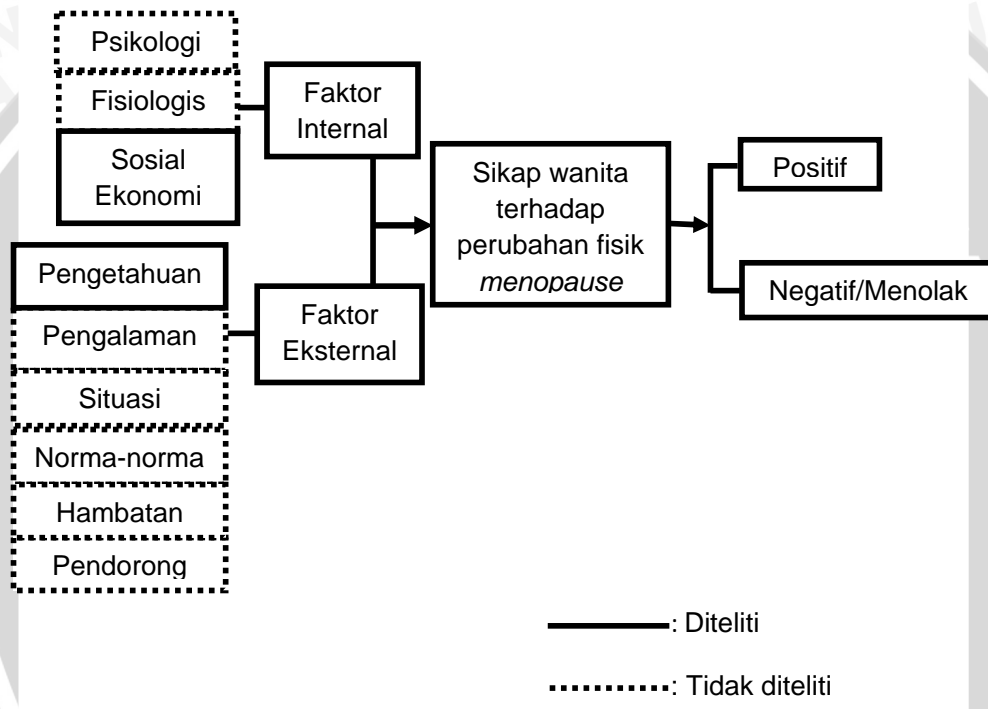
Gambar 3.1 Kerangka Konseptual
