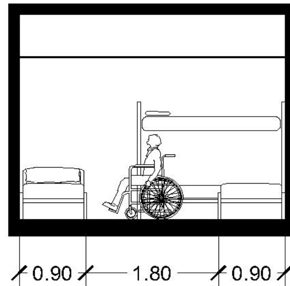
POT. KAMAR TIDUR E
