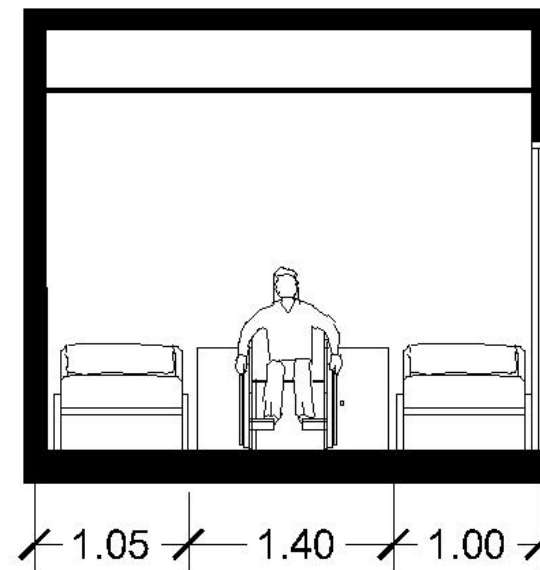
POT. KAMAR TIDUR C SKALA 1:50
