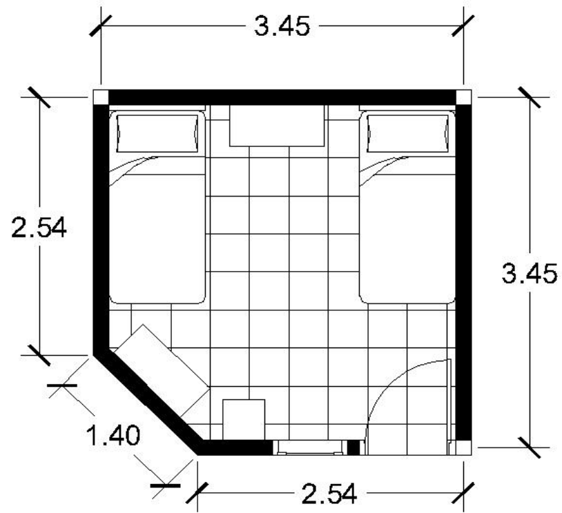
KAMAR TIDUR D SKALA 1:50
