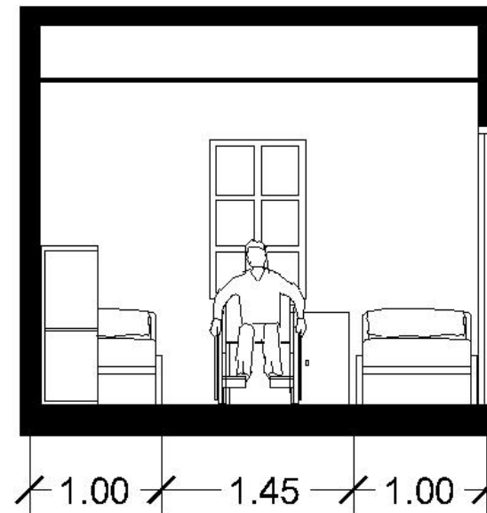
POT. KAMAR TIDUR A SKALA 1:50
