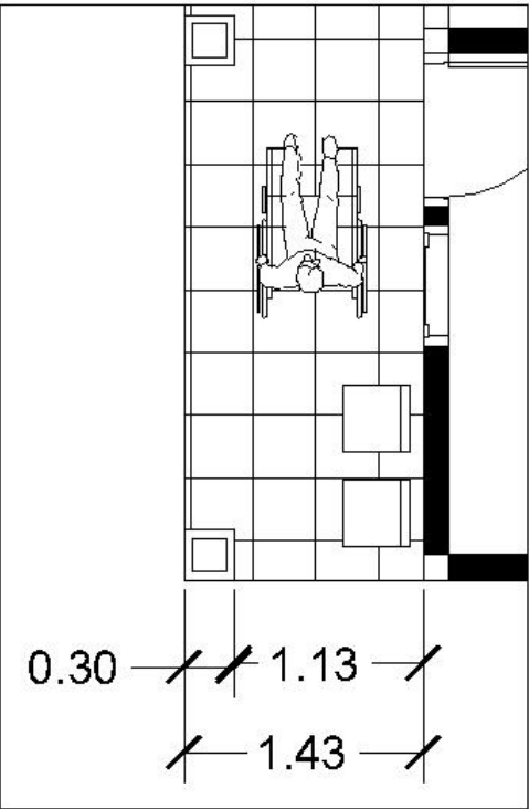
SELASAR A SKALA 1:50
