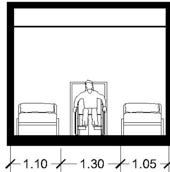
POT. KAMAR TIDUR D SKALA 1:50
