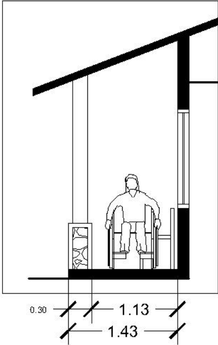
POT. SELASAR A SKALA 1:50
