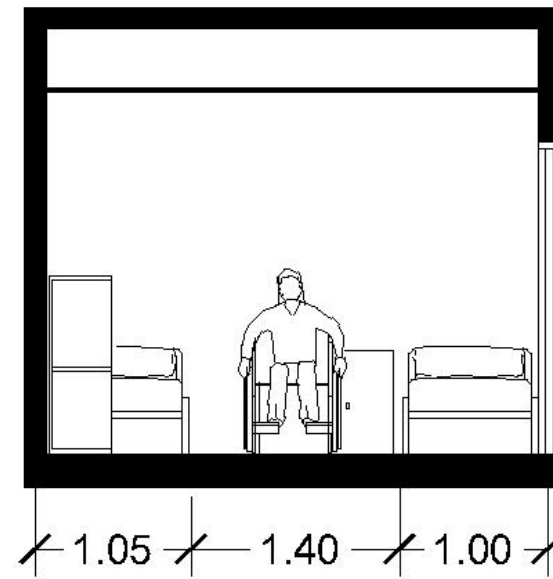
POT. KAMAR TIDUR B SKALA 1:50
